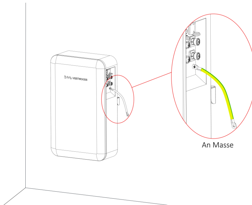
Abbildung 10. Erdung des V-Power S05
