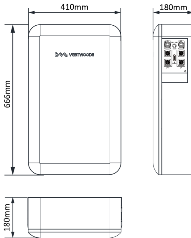
Abbildung 2. Abmessungen des V-Power S05 (Einheit: mm)
