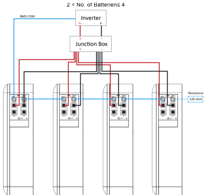
Abbildung 18. Anschließen der Kommunikationskabel ( 2 < \text{Batterien} \leq 4 )
