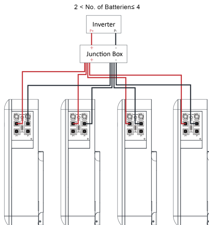
Abbildung 14. Anschließen der Stromkabel ( 2 < \text{Batteries} \leq 4 )
