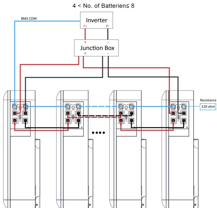
Abbildung 19. Anschließen der Kommunikationskabel ( 4 < \text{Batterien} \leq 8 )
