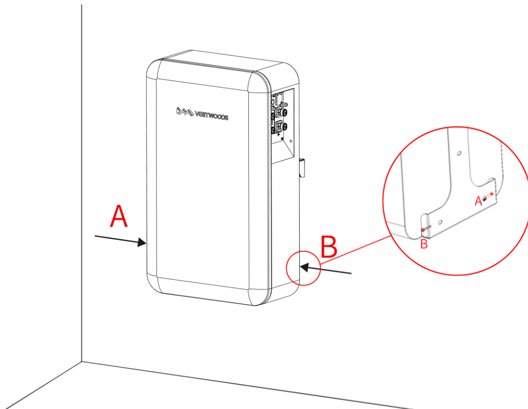
Abbildung 9. Montage von V-Power S05
